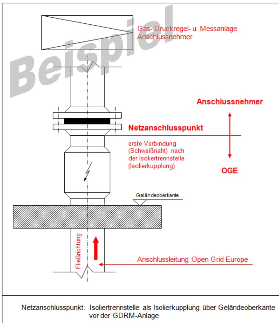
Abbildung 6: Prinzipskizze
