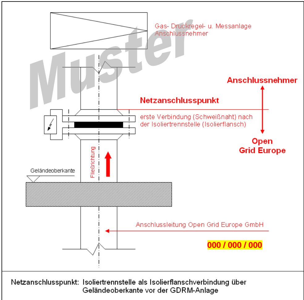
Abbildung 6: Prinzipskizze
