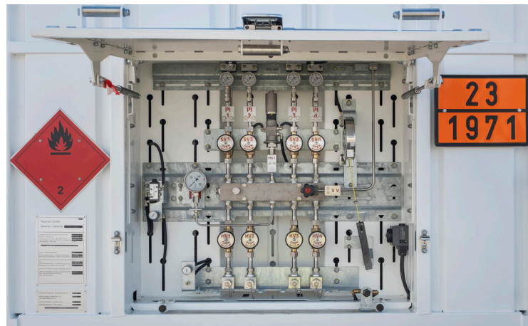
Anschlusspunkte CNG-Trailer
