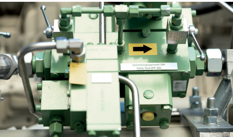
Sicherheitsabsperrentil (SAV)
