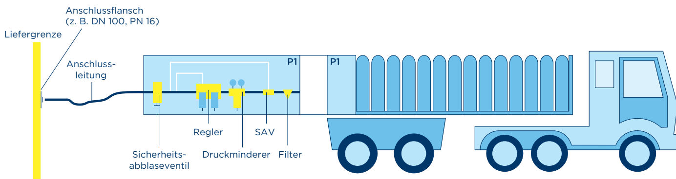
Mobile Erdgasversorgung im Betrieb
